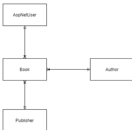
Slika 1. Primjer jednostavnog ER modela za evidenciju knjiga
